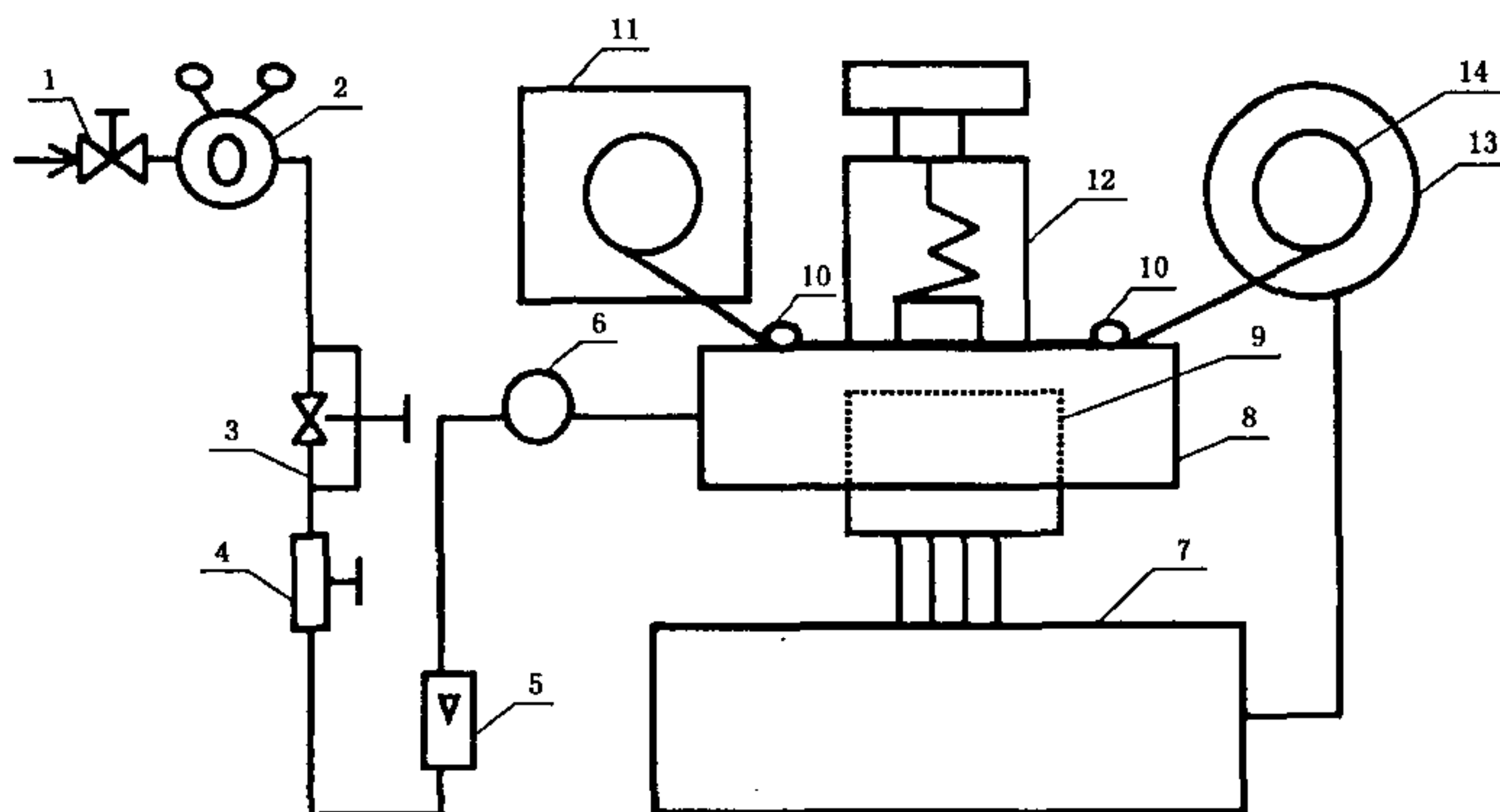
1—标准气或样品气入口开关阀；2—减压阀；3—稳压阀；4—稳流阀；5—转子流量计； 6—润湿器；7—数字处理系统；8—反应室；9—光电系统；10—导纸轮；11—密封盒； 12—压纸器；13—纸带；14—卷纸马达
